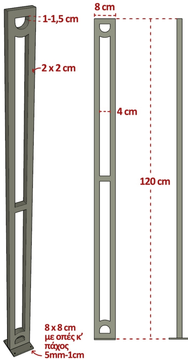
Εικόνα 1. Σχέδια νέου μεταλλικού ορθοστάτη
